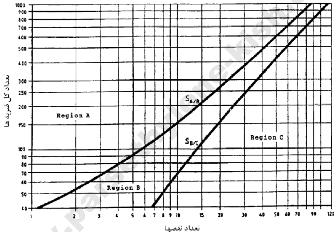
شکل ۳- تعداد نمونه ها برای ۱۰ درصد TIR (در ۹۰ درصد درجه اطمینان)
